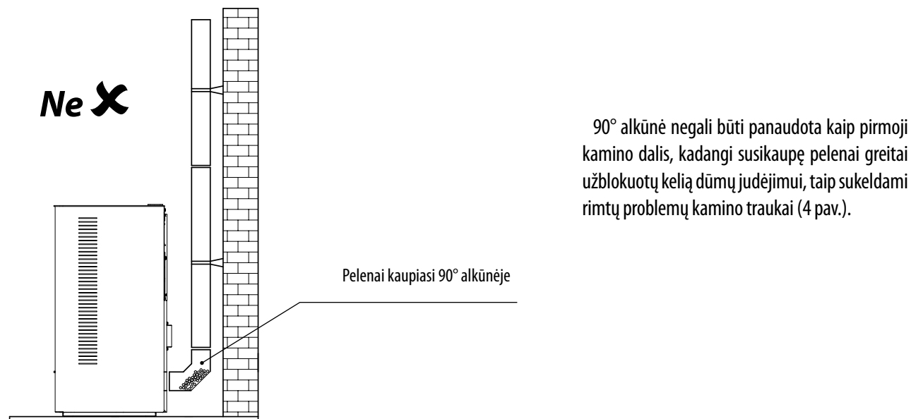
4 pav. Neteisingas montavimas panaudojant 90° alkūnę kaip pirmąjį elementą.
