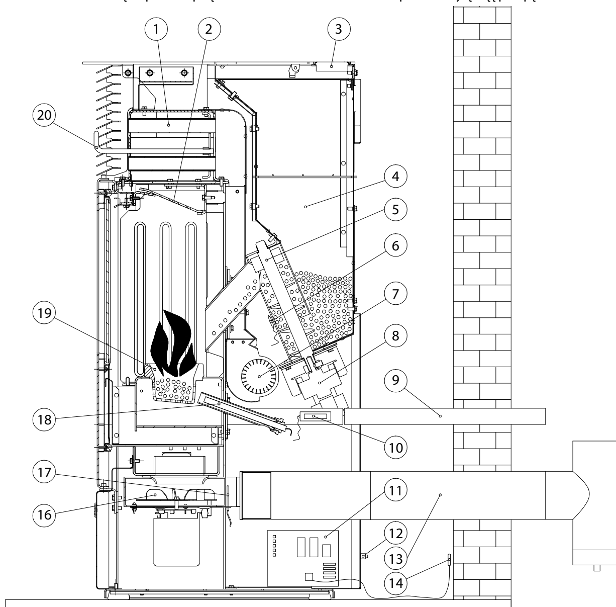
1 pav. Konstrukciniai krosnelės elementai
