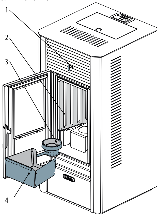
12 pav. Dažniausiai tikrinami elementai ir jų vietos.
