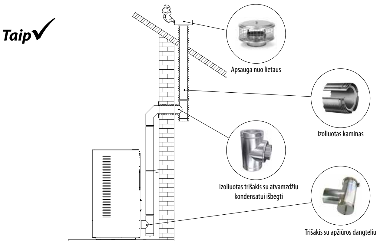
8 pav. Montavimas su vidiniu/išoriniu kaminiu.
